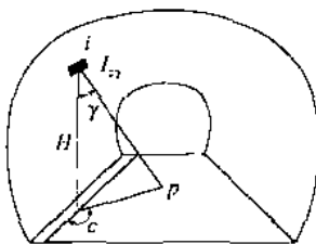
图 10-1 灯具光强示意图
