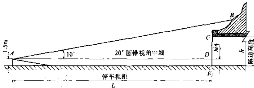
图 4-1 洞外亮度 L_{20}(S) 测试示意图
