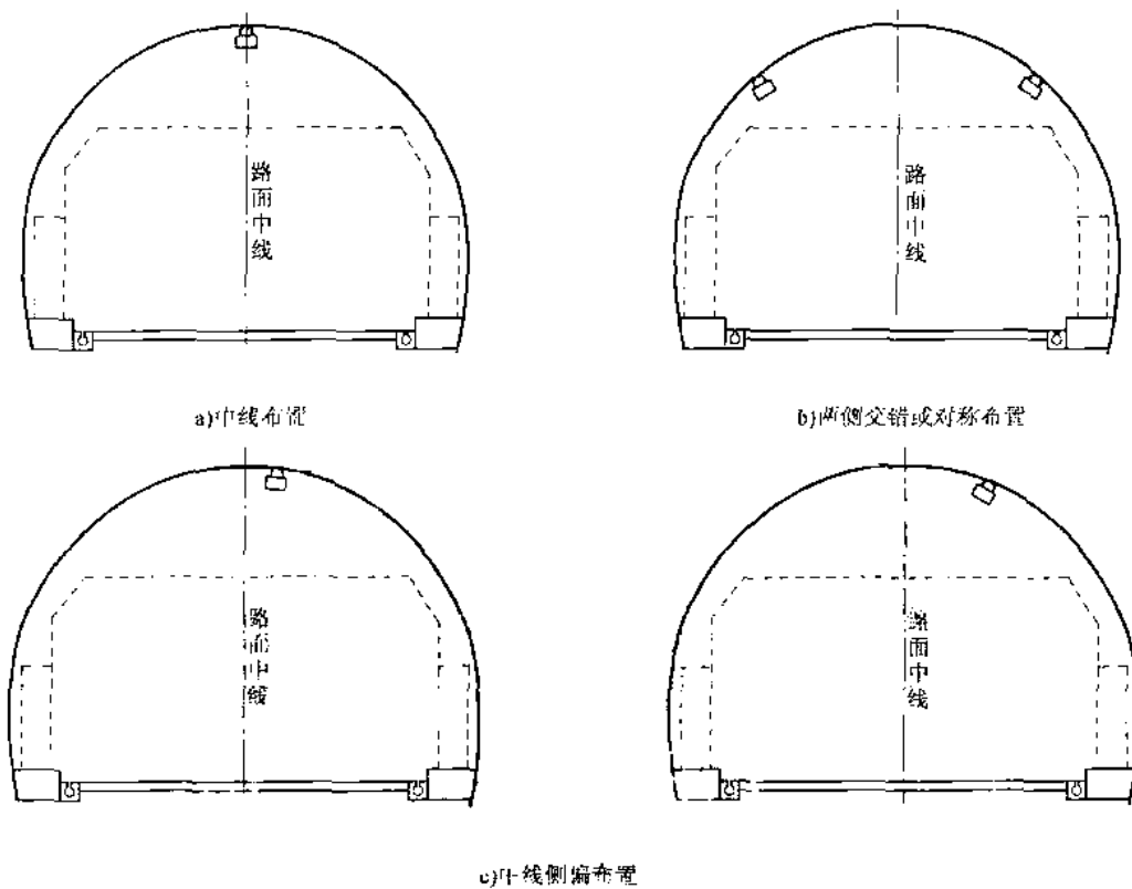
图 3-1 灯具布置形式示意图
