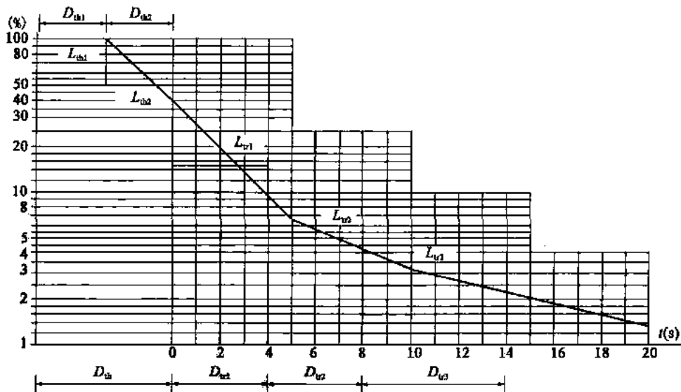
图 5-1 过渡段长度与相应亮度
