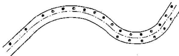
图6.2.4-2 反向曲线段上的灯具布置示意图
