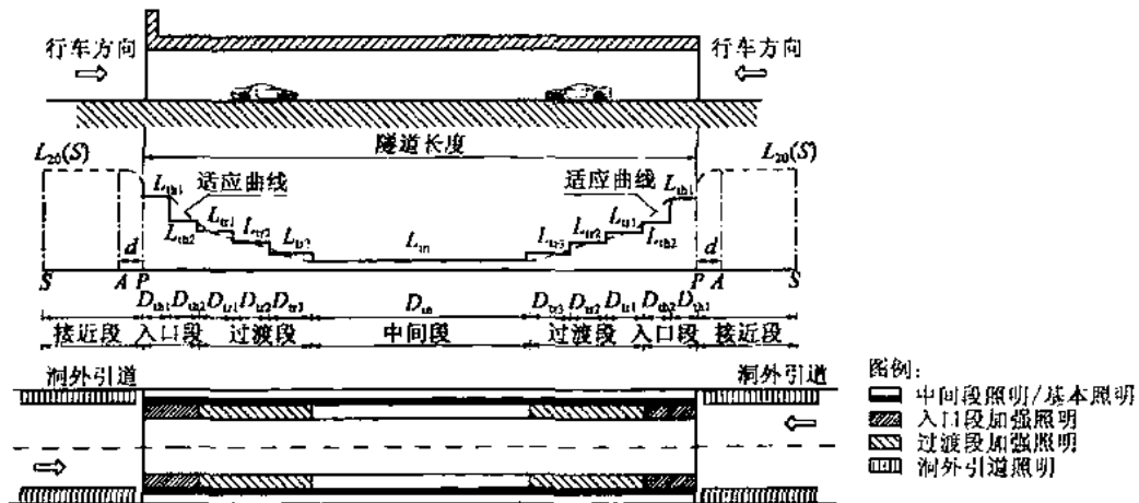
图 3.0.6 双向交通隧道照明系统分段图
