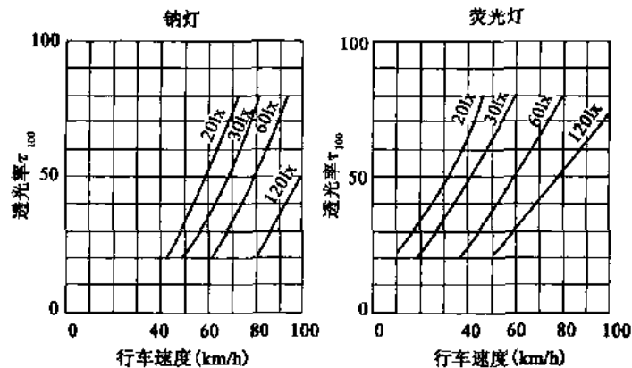
图 9-1 透过率、车速、照度和光源之间的关系
