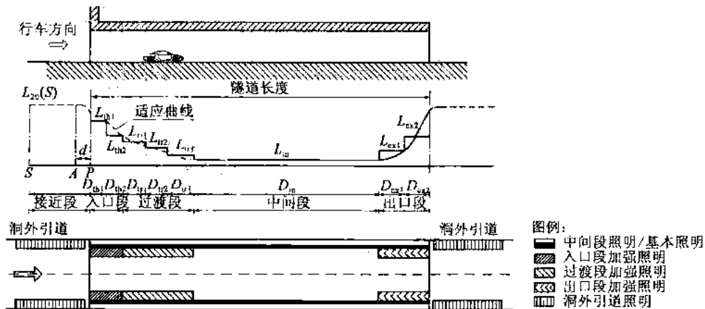
图 3.0.5 单向交通隧道照明系统分段图
