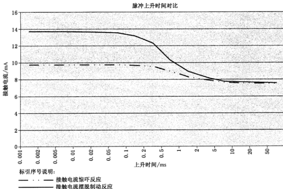
图 H.5 接触电流与上升时间点状图, 20 ms 方波
