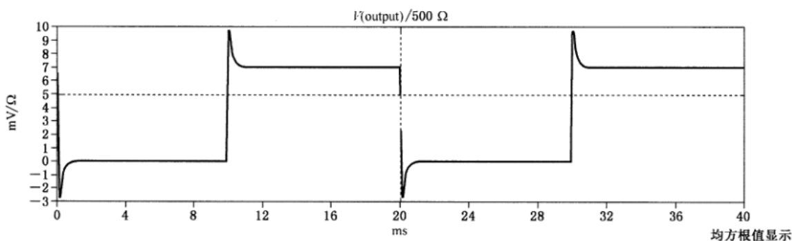
图 H.8 50 Hz 方波,0.1 ms 上升时间,摆脱制动
