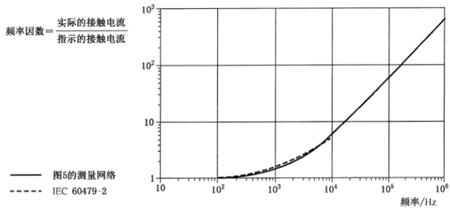
图 F.3 摆脱制动电流的频率因数
