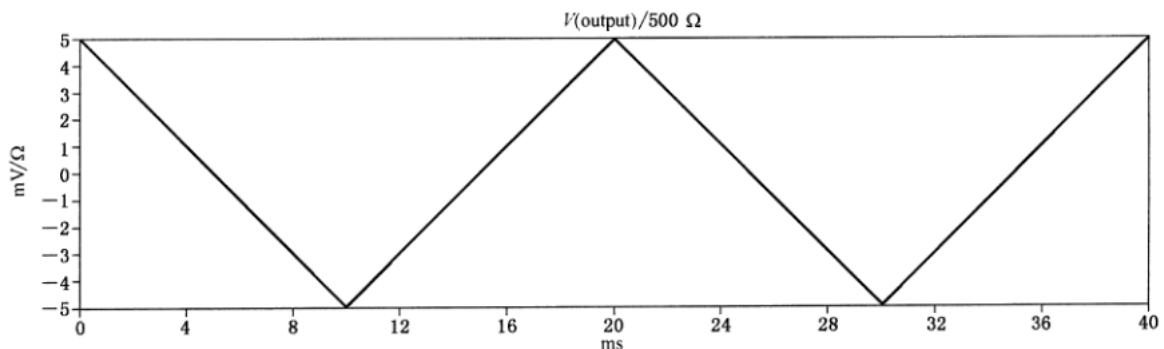
图 H.1 三角波形接触电流,惊吓反应
