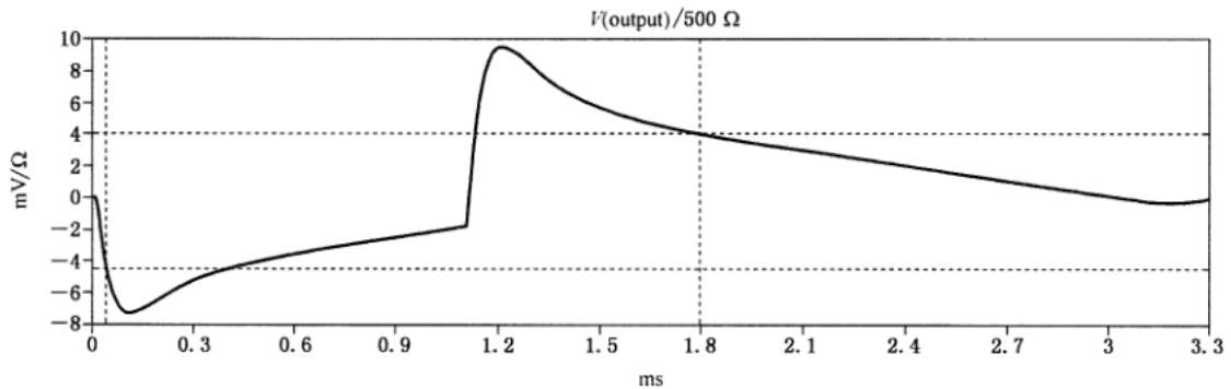
图 H.11 显示有效值窗口
