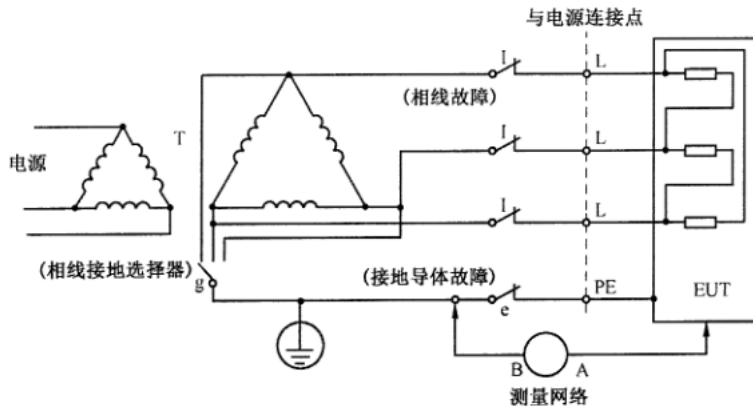
图 13 接到未接地的三角形配电系统的三相设备的试验配置
