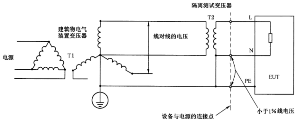
图 2 带有隔离变压器的接地中线
