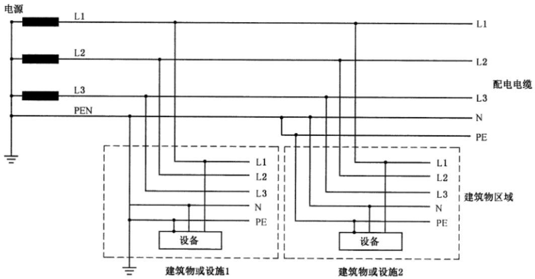
图 I.2 TN-C-S 配电系统实例
