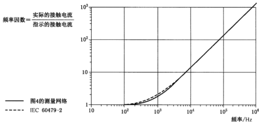
图 F.2 感知电流/惊吓反应电流的频率因数
