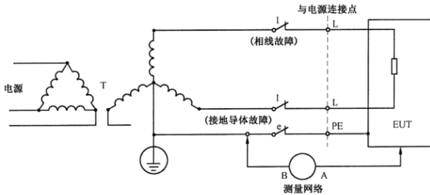
图 8 接到星形 TN 或 TT 系统的相间的单相设备的试验配置
