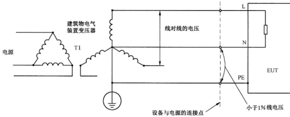
图 1 直接供电的接地中线
