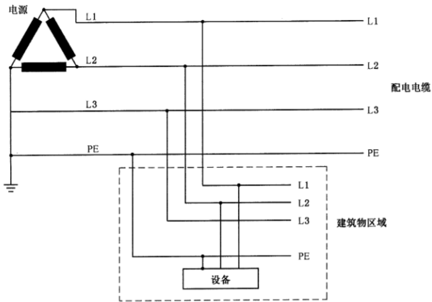
接地的相线
