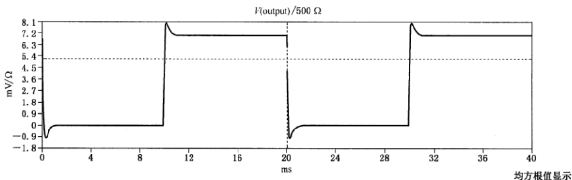
图 H.7 50 Hz 方波,0.1 ms 上升时间,惊吓反应
