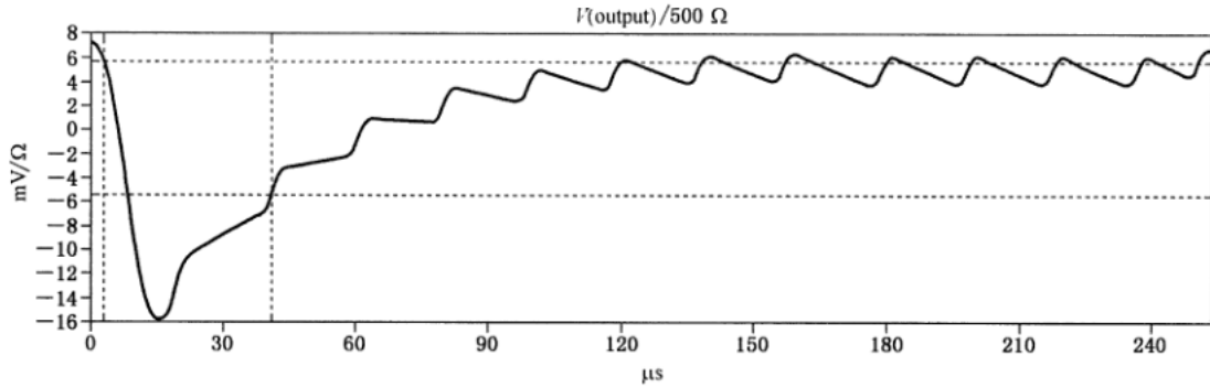
图 H.10 显示有效值窗口
