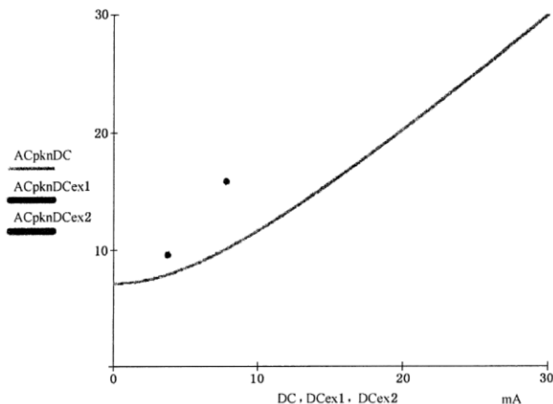
图 H.9 IEC 60479-2 AC+DC 组合(增强额外数据)的摆脱阈值
