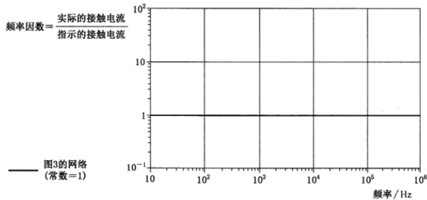
图 F.1 电灼伤电流的频率因数
