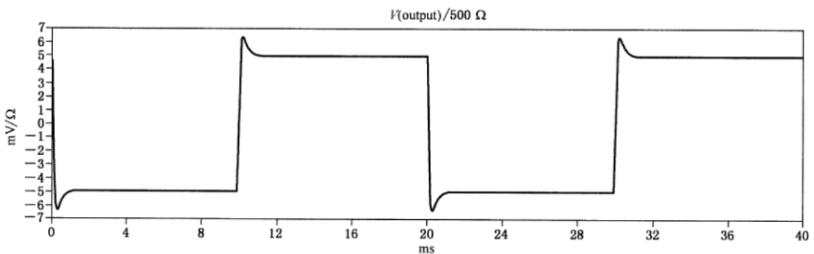
图 H.3 1 ms 脉冲响应, 惊吓反应
