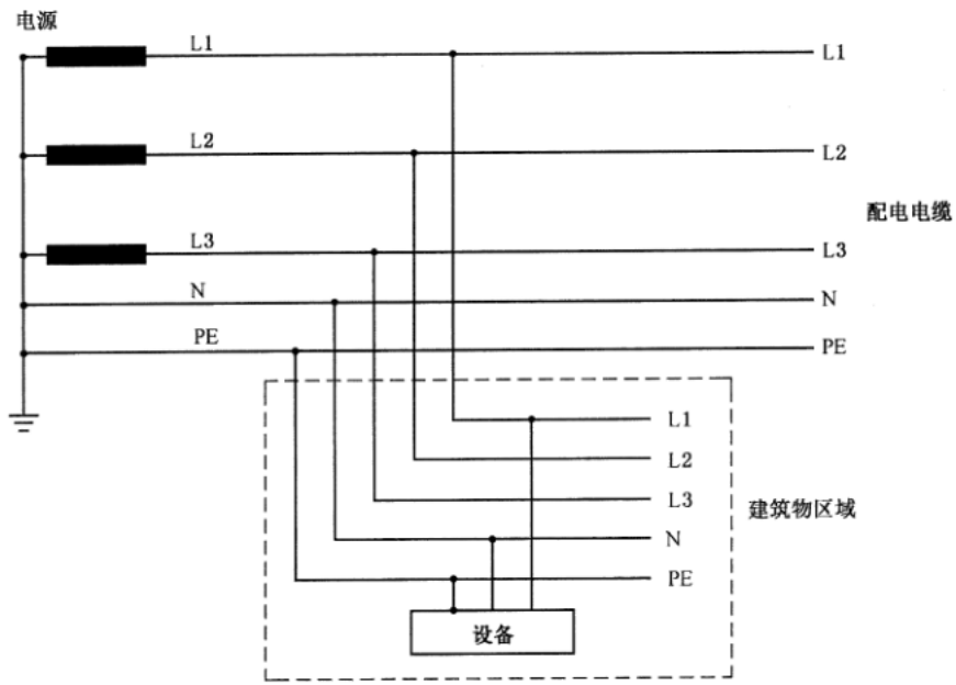
单独的中线和保护接地线
