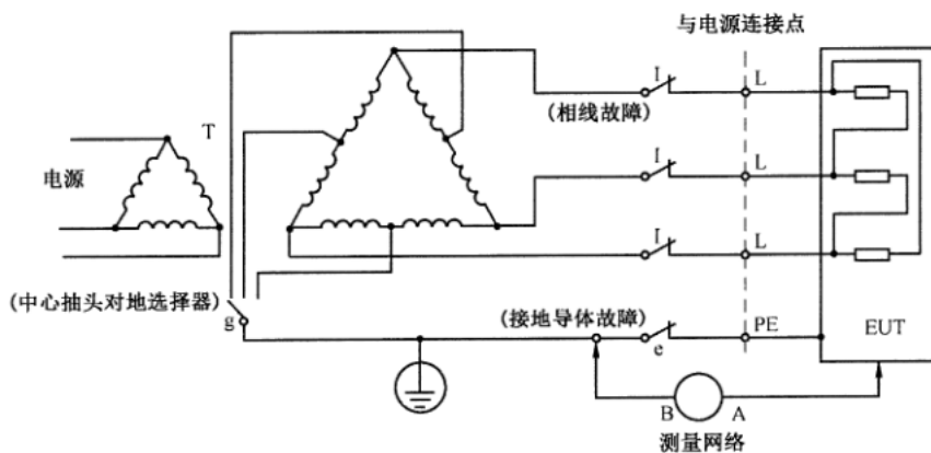
图 13 接到未接地的三角形配电系统的三相设备的试验配置
