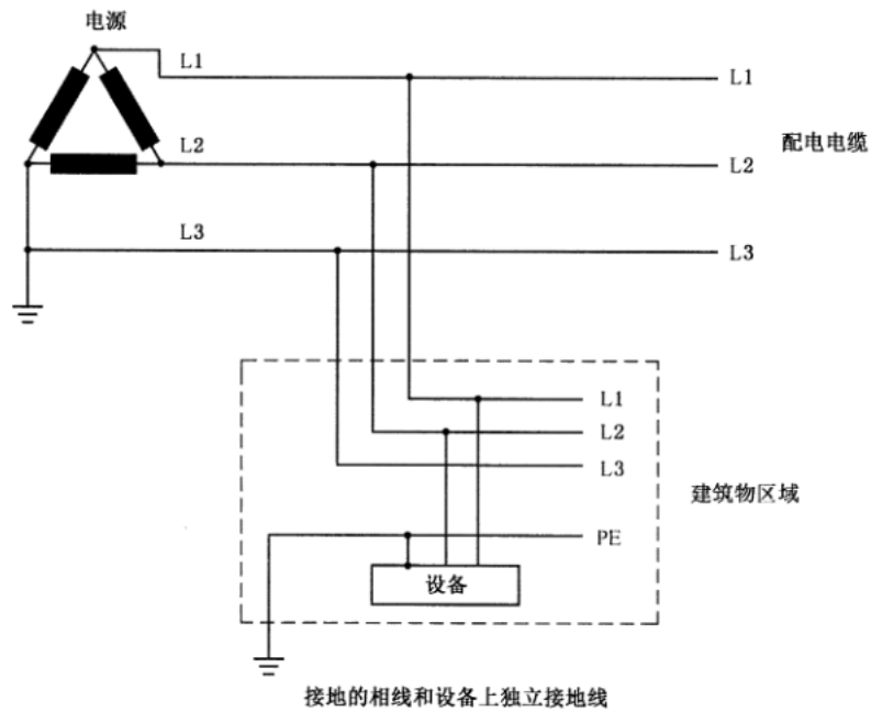
图 I.6 三相线的 TT 配电系统
