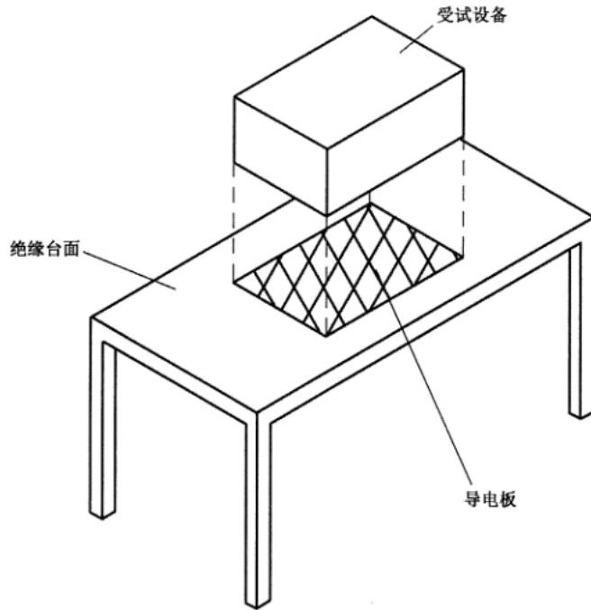
图 B.1 设备试验台
