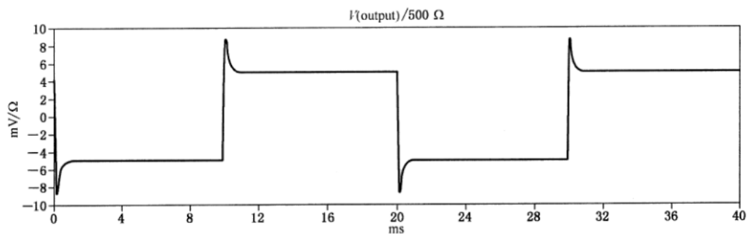
图 H.4 1 ms 脉冲响应, 摆脱制动
