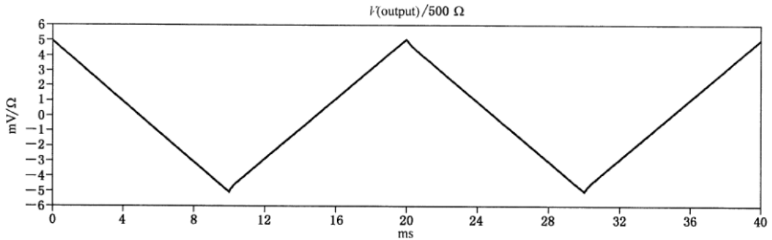
图 H.2 三角波形接触电流, 摆脱制动反应
