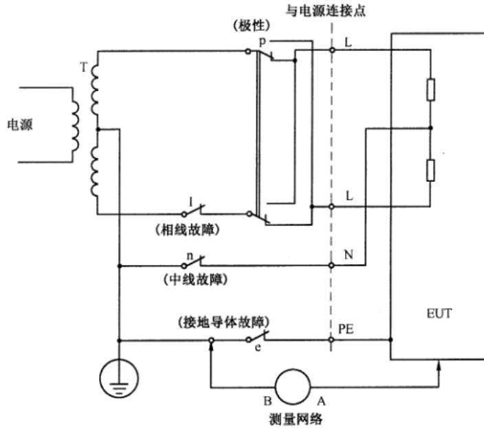
图 6 接到星形 TN 或 TT 系统的单相设备的试验配置
