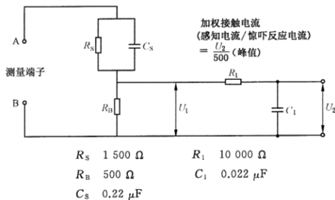
图4 加权接触电流(感知电流或惊吓反应电流)的测量网络
