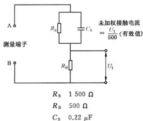
图3 未加权的接触电流的测量网络
