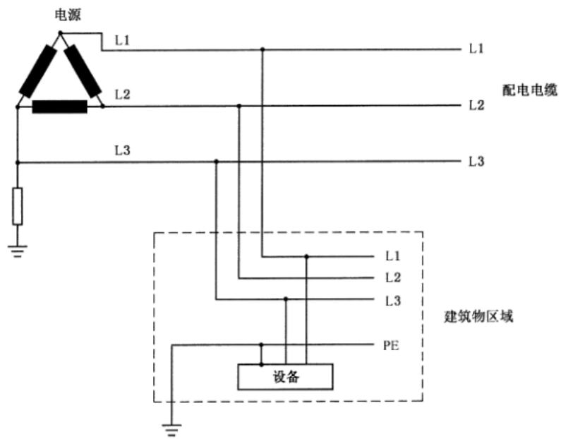
图 I.8 三相线 IT 配电系统实例
