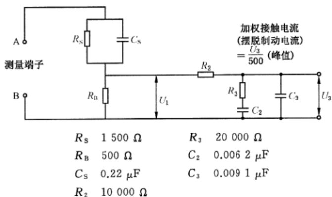
图5 加权接触电流(摆脱制动电流)的测量网络
