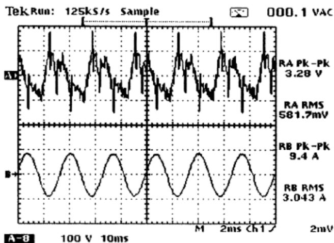
图 H.6 PFC 开关电源接触电流波形
